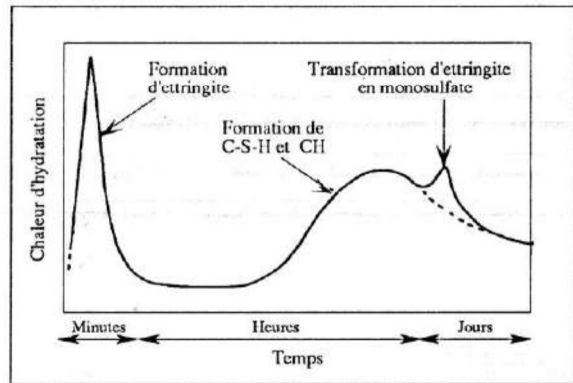
Figure 3 : Représentation schématique de la réaction d'hydratation des ciments Portland [6].
