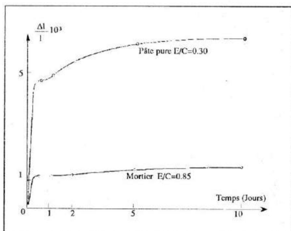
Figure 10 : Variations dimensionnelles comparées de pâtes pures et mortiers [4].
