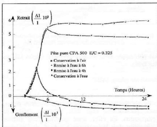
Figure 6 : Réversibilité des déformations de retrait [4].
