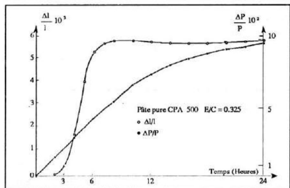
Figure 4 et 5 : Retrait et pertes de poids au cours des 24 premières heures [4].
