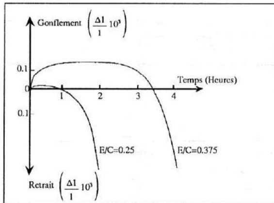
Figure 2 : Variations dimensionnelles instantanées [4].
