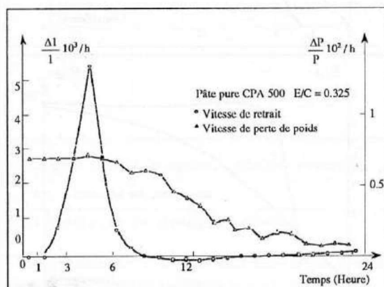
Figure 7 : Evolution des vitesses de retrait et de pertes en poids [4].
