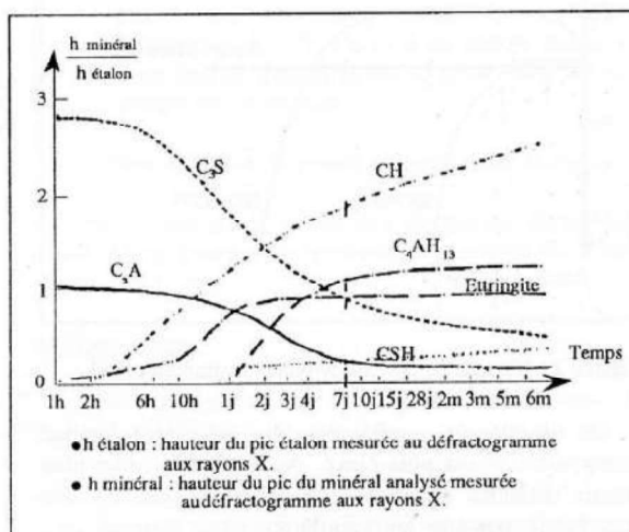
Figure 8 : Variation des constituants anhydres et hydratés du ciment Portland en fonction du temps [7].
