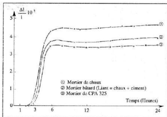
Figure 9 : Influence de la nature du liant [4].
