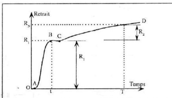
Figure 1 : Allure générale des variations dimensionnelles des mortiers [4].
